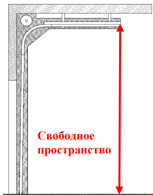
Высокий монтаж
