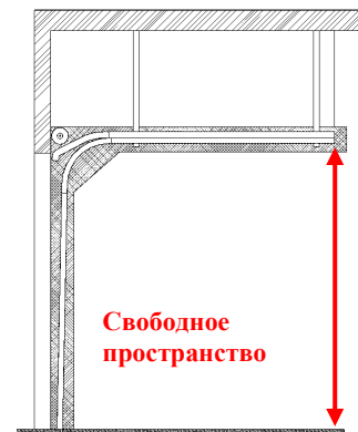
Стандартный монтаж
